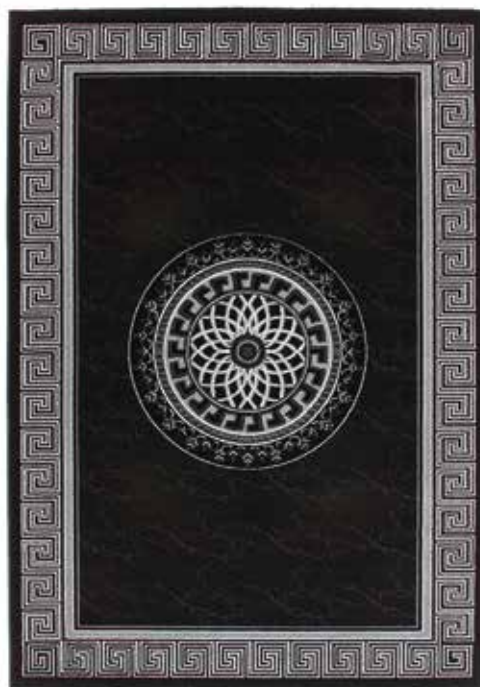
ARA 776 Black
